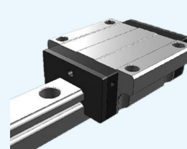
Bauart EM / Type EM Wagenanschluss: Gewindebohrung / Durchgangsbohrung Mounting method: Tapped hole / through hole
