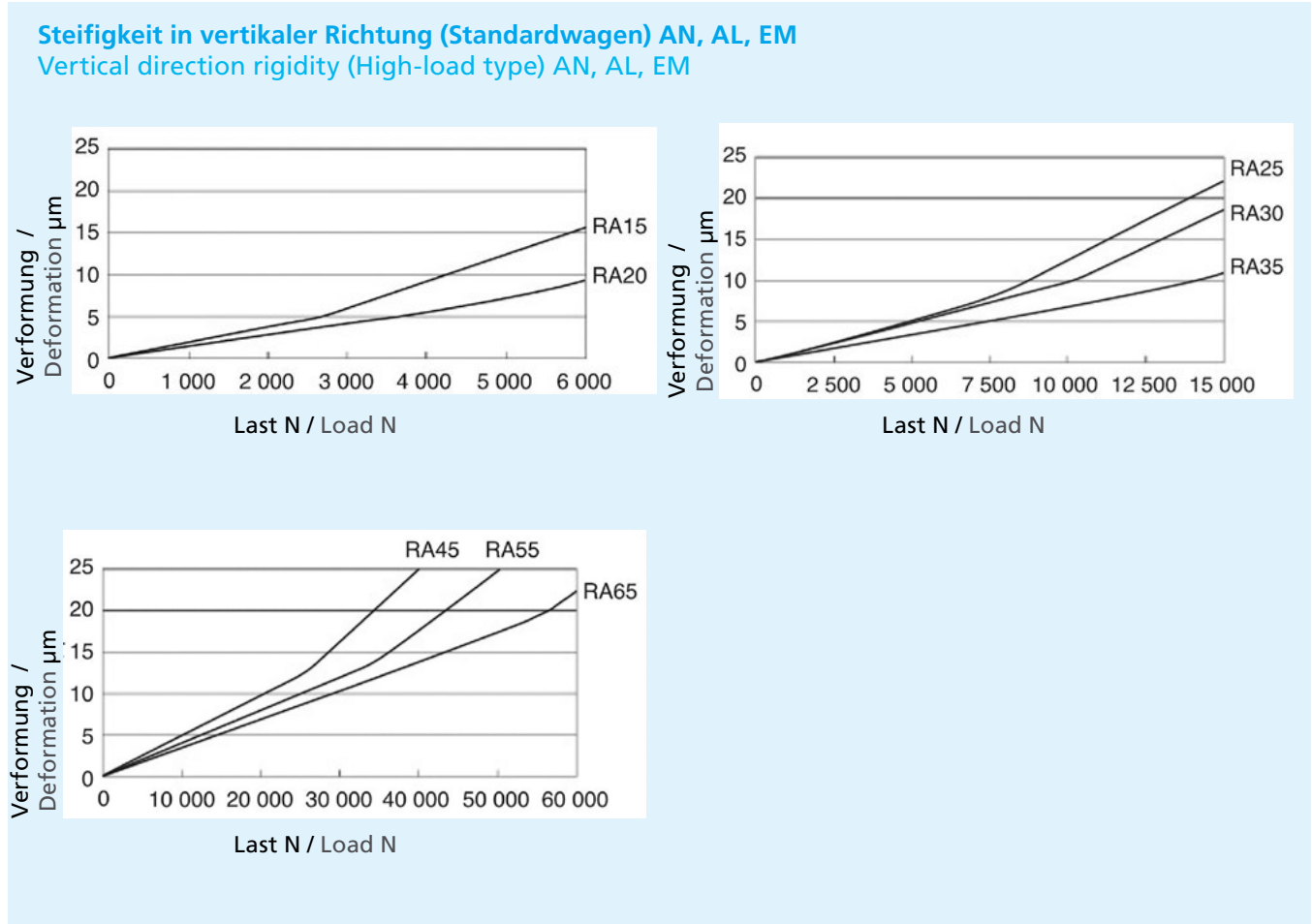
Abb. 5 Steifigkeit der mittleren Vorspannung
